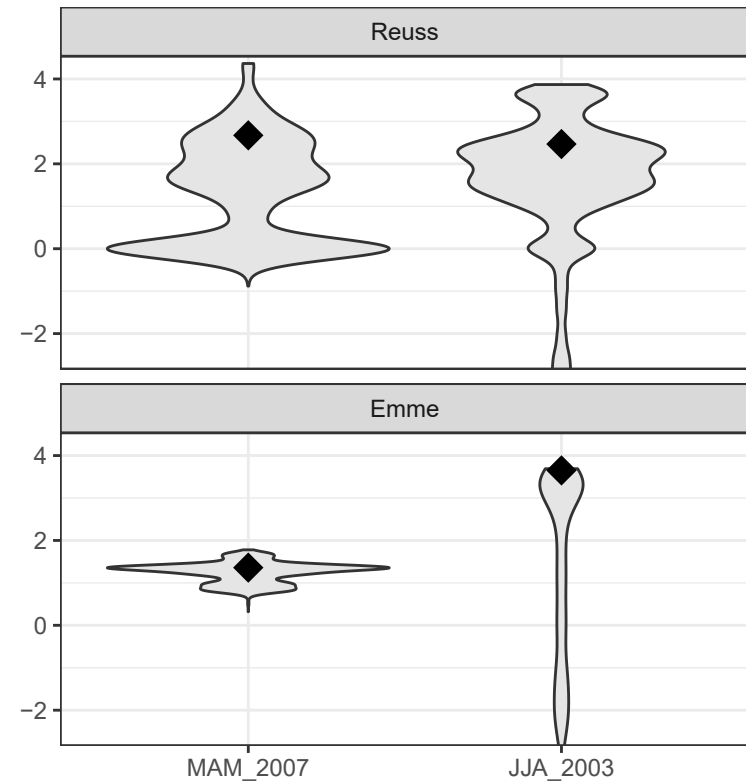
(b) Actual evapotranspiration anomalies
