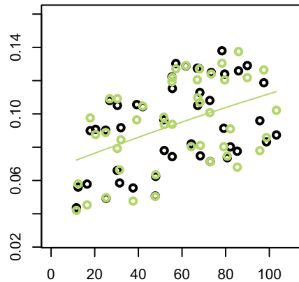
R-vine copula
