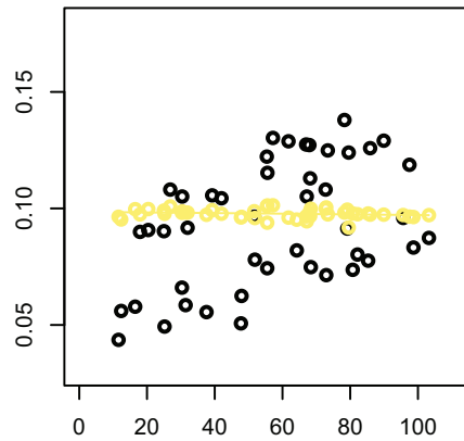
R-vine copula
