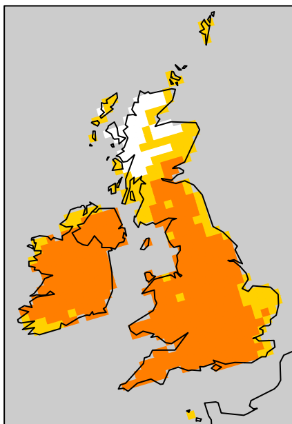
(c) EOF 3 (6 %)
