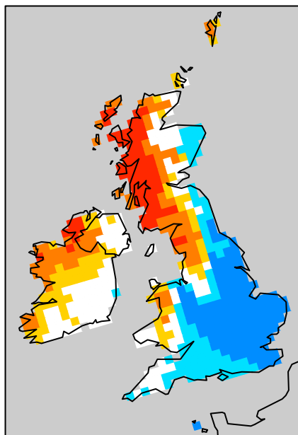
(d) EOF 4 (5 %)
