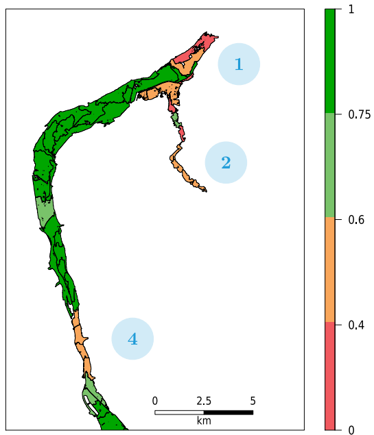
(b) CSI
