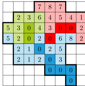
(d) HAND value
