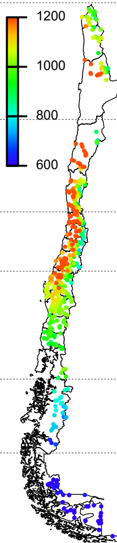
(d) Mean annual PET (mm)
