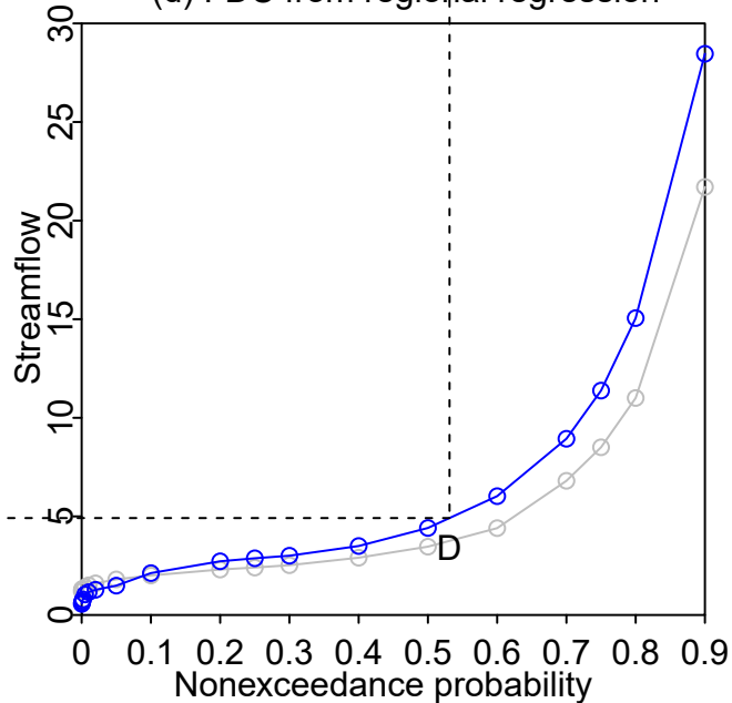
(d) FDC from regional regression
