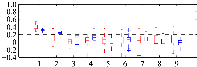
(h) MHRB-DJF
