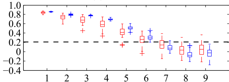
(d) UHRB-DJF
