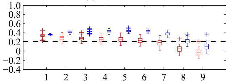
(b) UHRB-JJA
