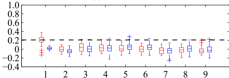
(g) MHRB-SON
