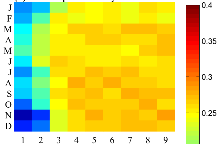
(d) MHRB-forecast skill
