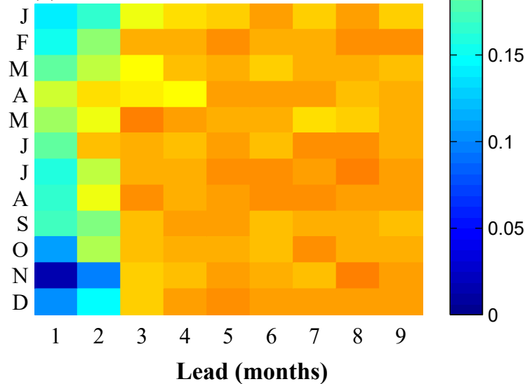
(d) MHRB-forecast skill
