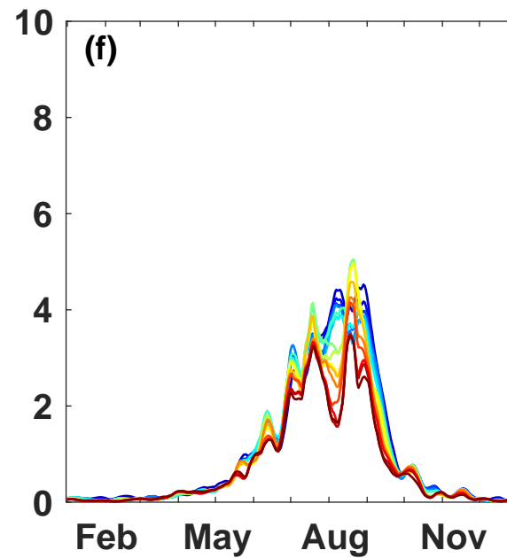
TVP - HyMOD
