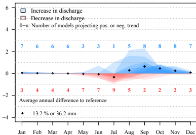
(d) RCP 8.5 (2070–2099)
