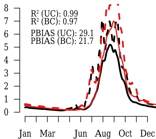
NorESM1-RCA4
