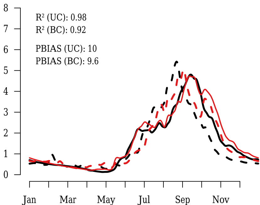
GFDL
