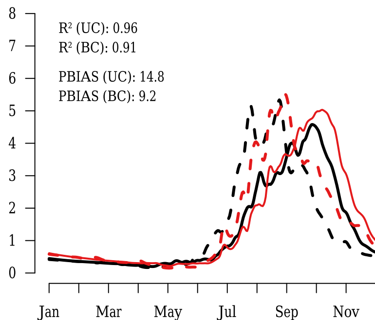
MIROC
