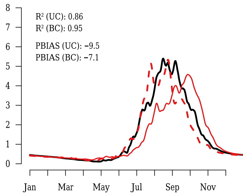
MIROC
