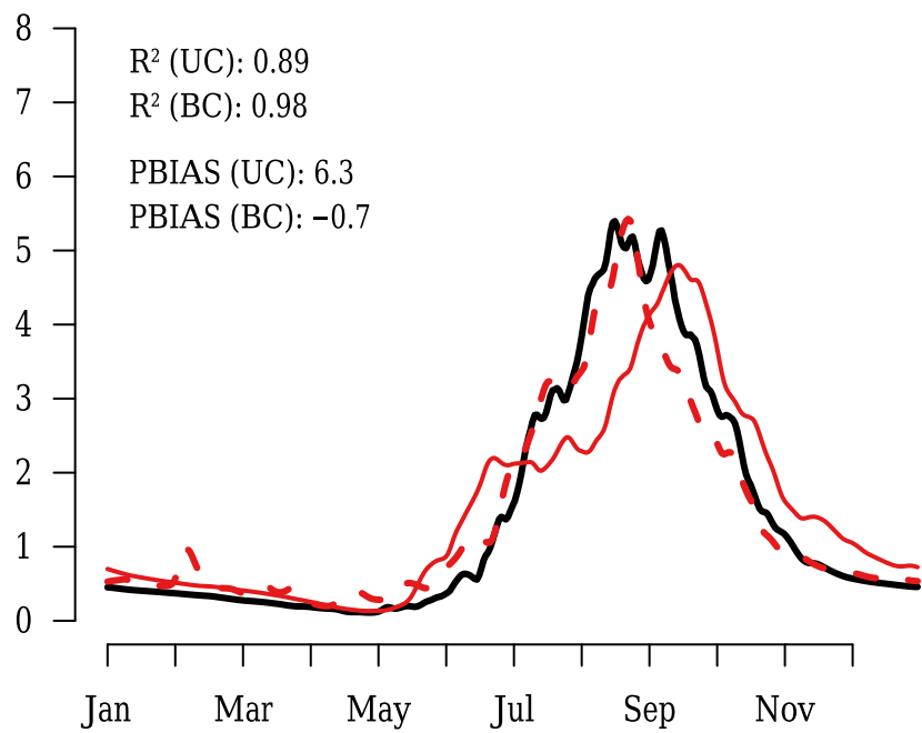
GFDL
