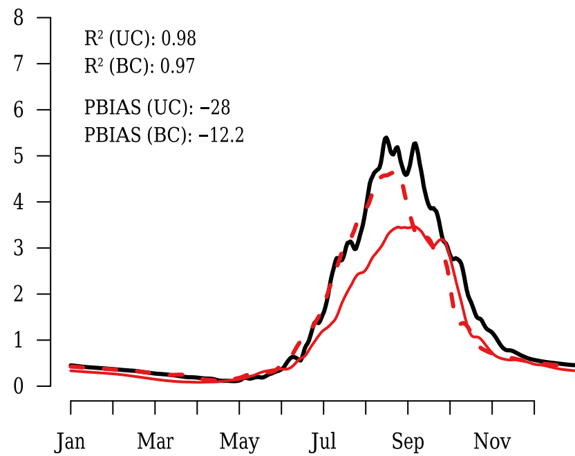
HadGEM
