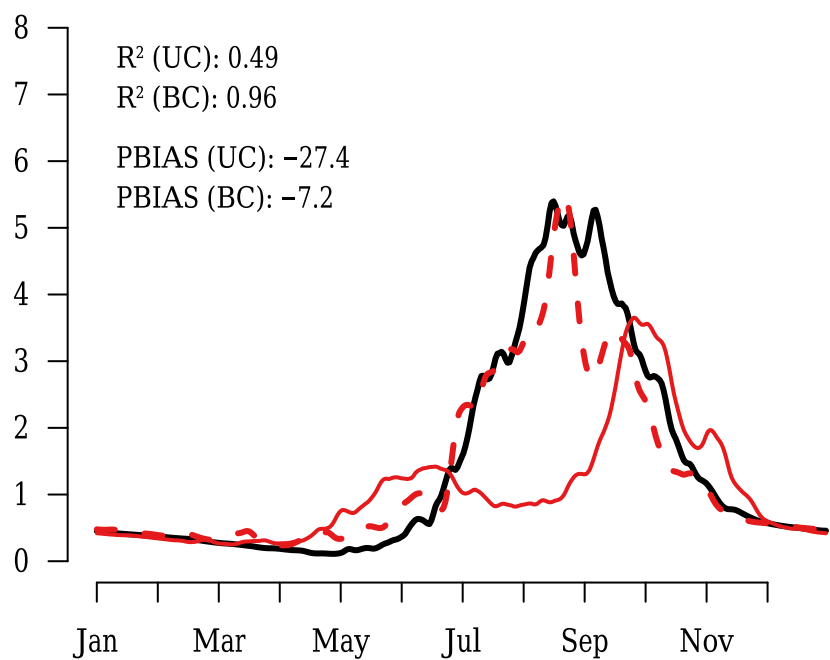
NorESM
