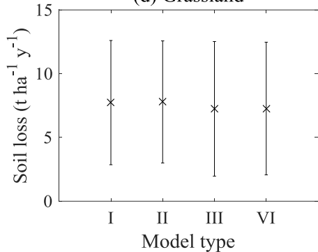
(d) Grassland
