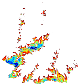
rcp85
