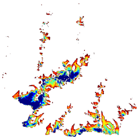
rcp26
