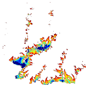
rcp45
