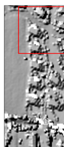
(b) Lidar DEM overview (2 m pixel −1 )
